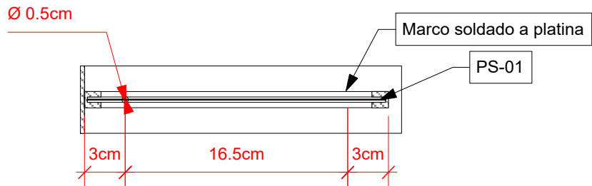
C Corte Horizontal Scale: 1:4
