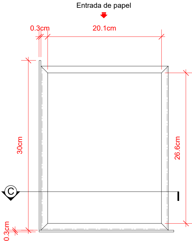
2 Vista Frontal Scale: 1:4
