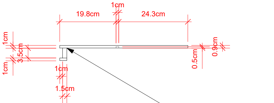
4 Vista Lateral Scale: 1:8
