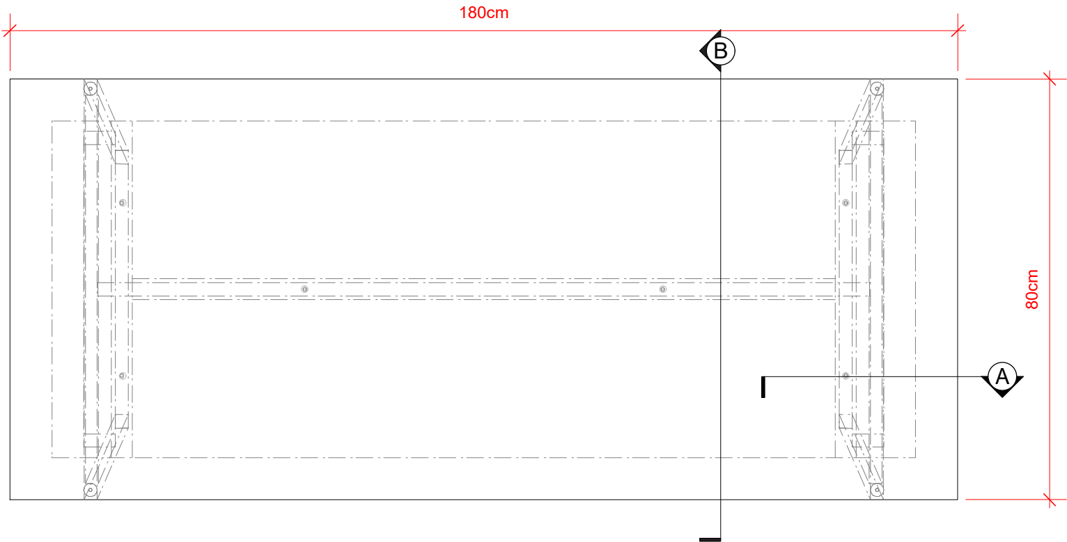
1 Vista Superior Scale: 1:10
