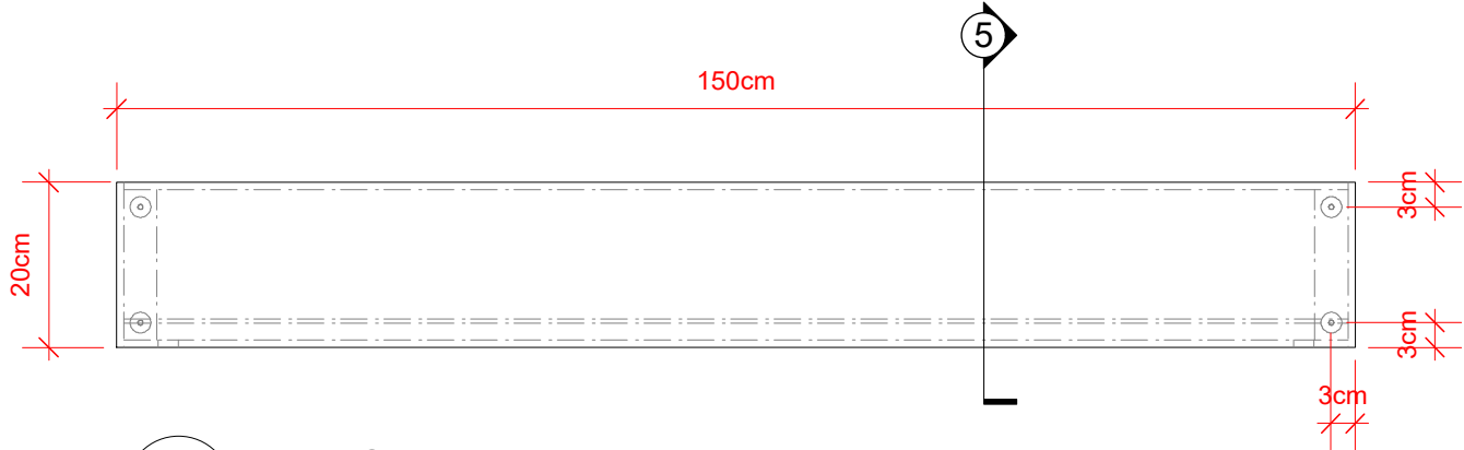
1 Vista Superior Scale: 1:10
