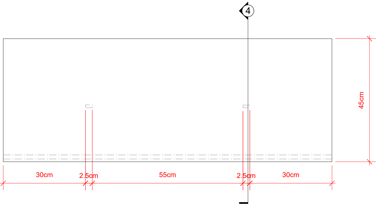
1 Vista Superior Scale: 1:8
