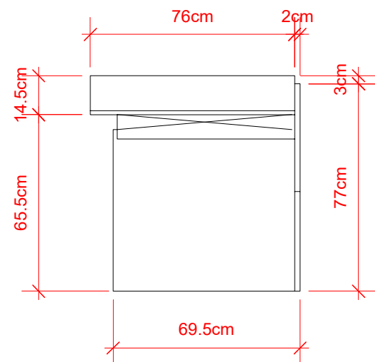
1 Vista Superior Scale: 1:20
