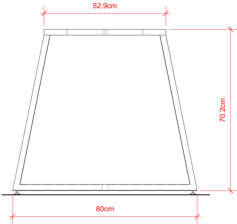
4 Vista Lateral Scale: 1:10
