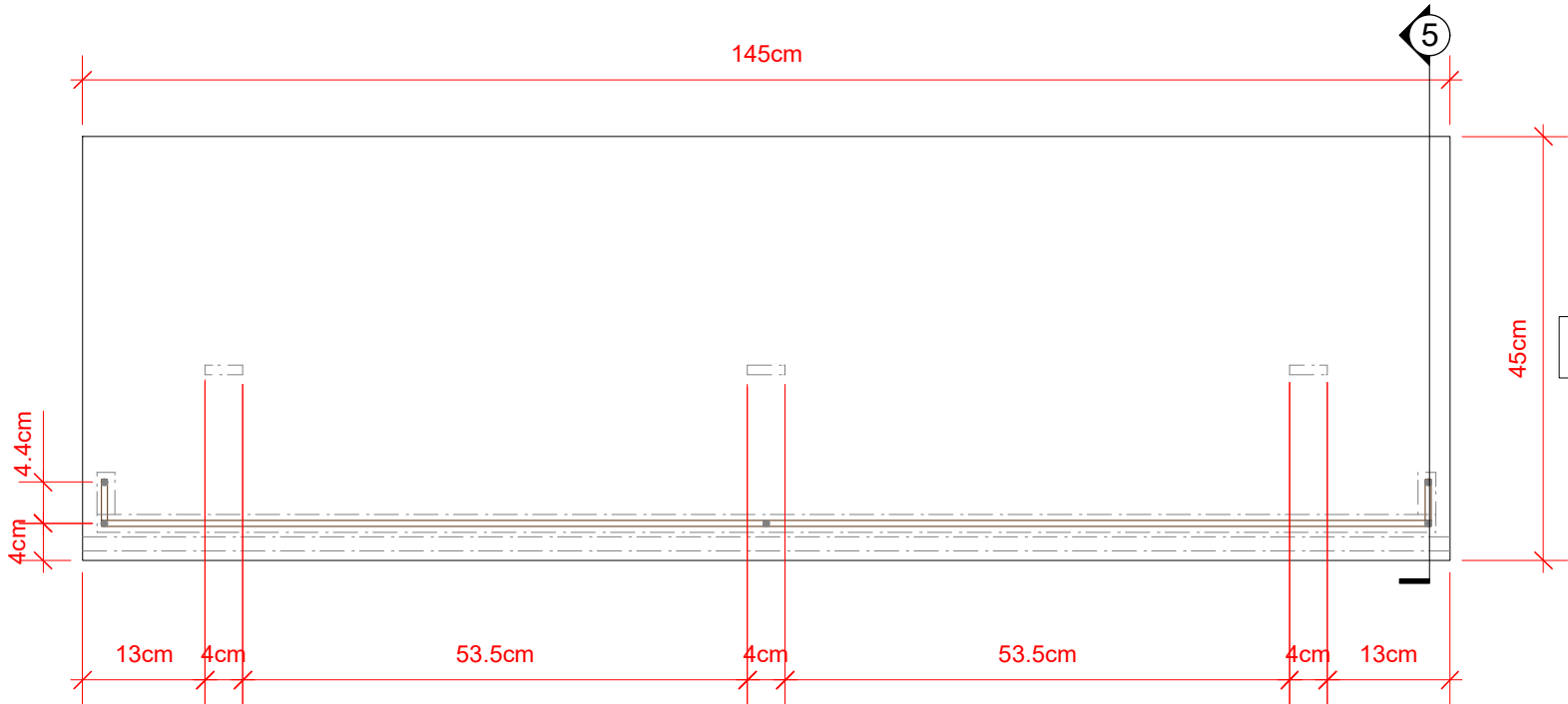
1 Vista Superior Scale: 1:8
