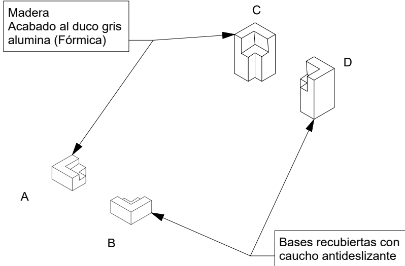
7 Isométrico Scale: 1:20
