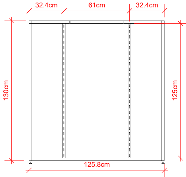
3 Estructura Cremallera Scale: 1:20
