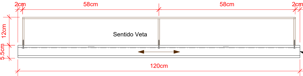
2 Vista Frontal Scale: 1:8
