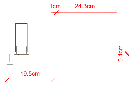
4 Vista Lateral Scale: 1:8
