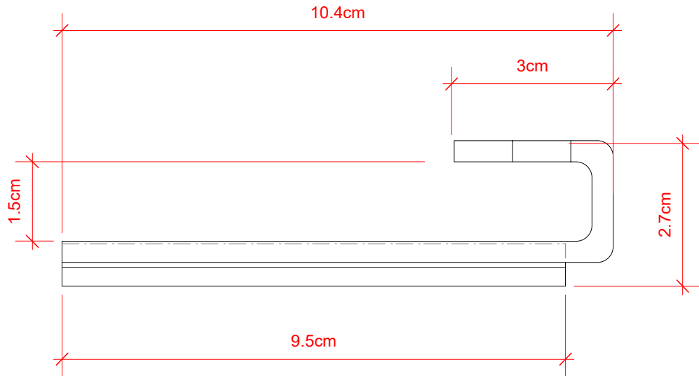
1 Vista Superior Scale 1:1
