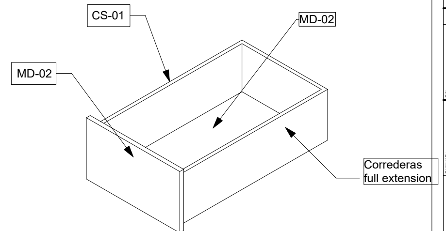
7 Isométrico Scale: 1:10
