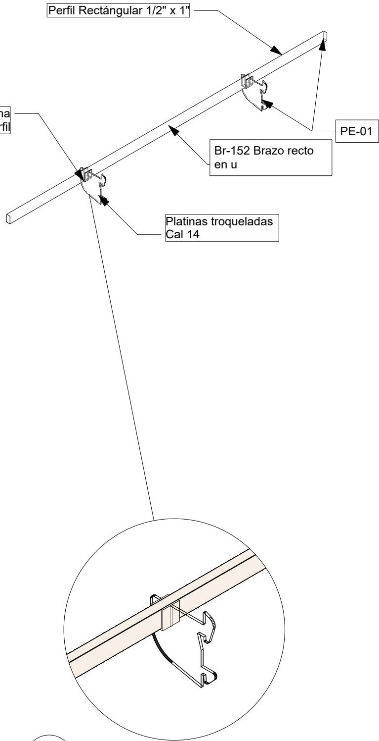
5 Detalle Scale: 1:4
