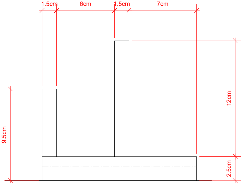
3 Isométrico Scale 1:2
