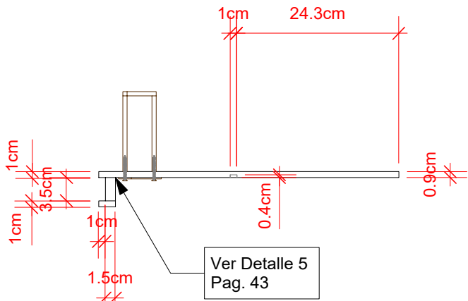
4 Vista Lateral Scale: 1:8
