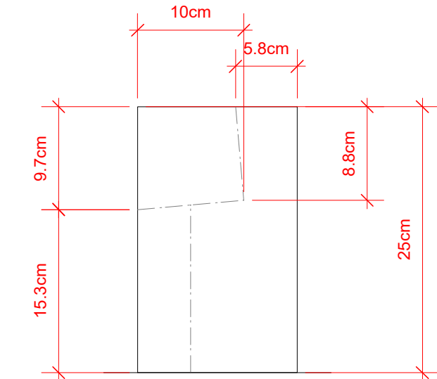
6 Vista Lateral Scale: 1:5
