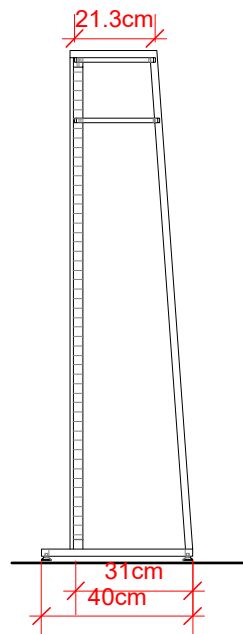
5 Vista Lateral Scale: 1:20
