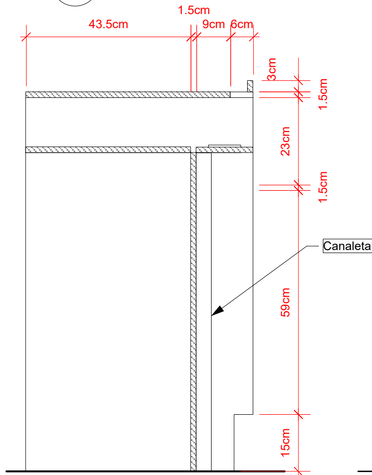
1 Corte A Scale: 1:10
