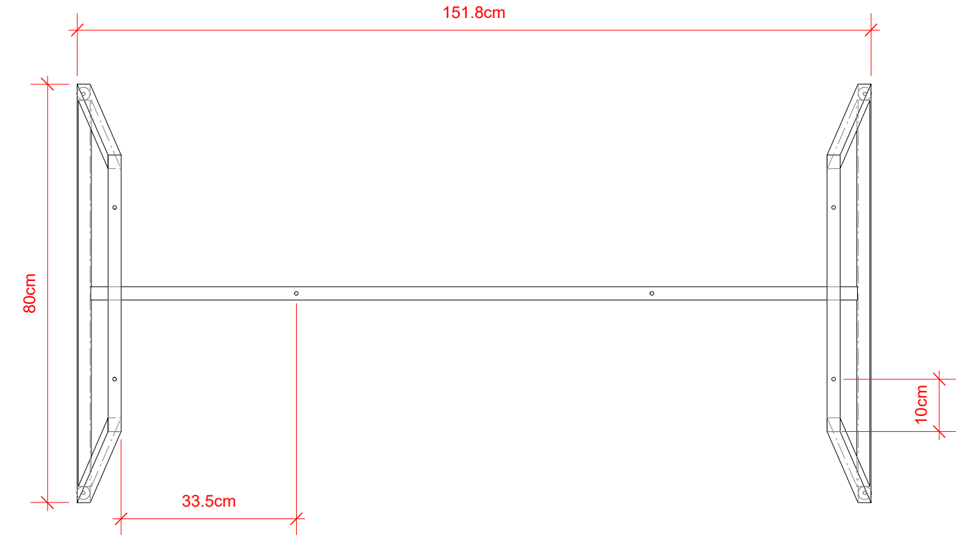
1 Vista Superior Scale: 1:10
