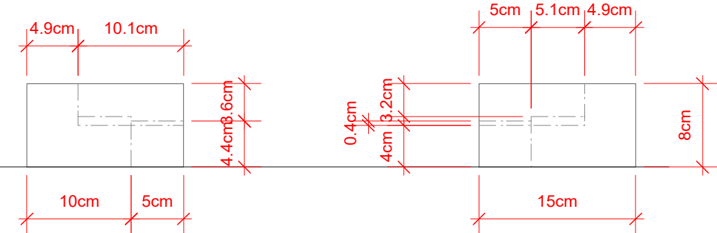
2 Vista Frontal Scale: 1:5
