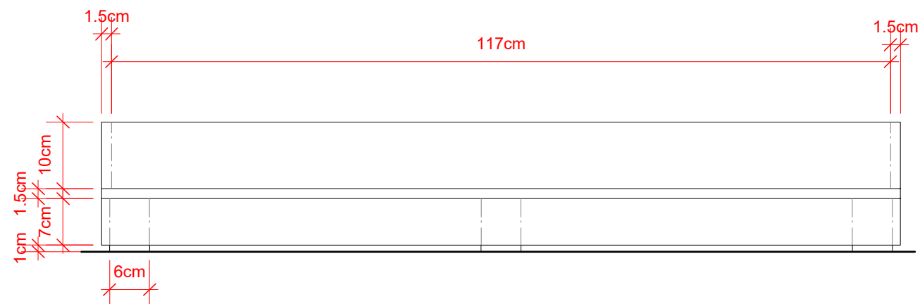
2 Vista Lateral Scale: 1:8
