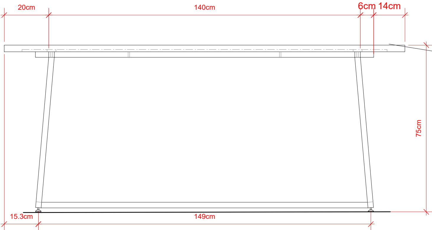
2 Vista Frontal Scale: 1:10
