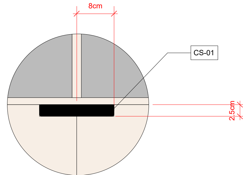
4 Detalle manijas puertas Scale: 1:5
