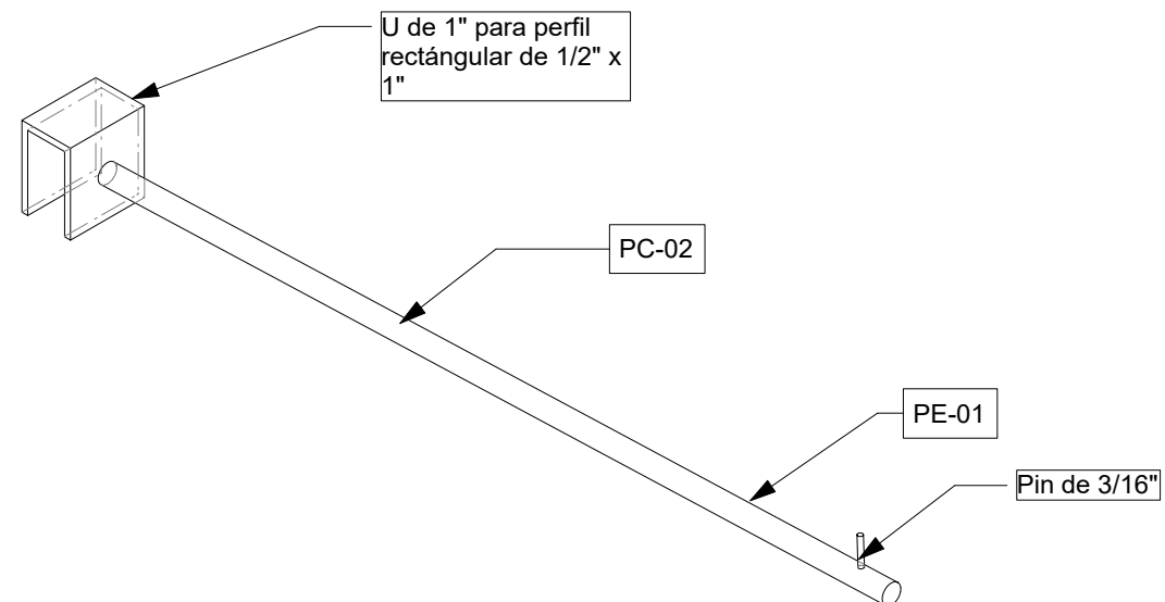
3 Isométrica Scale 1:2
