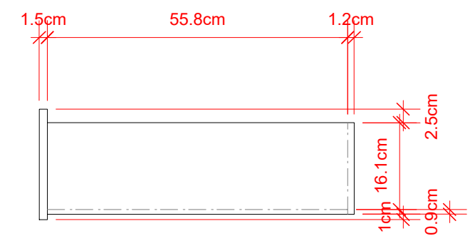
8 Vista Lateral Scale: 1:10
