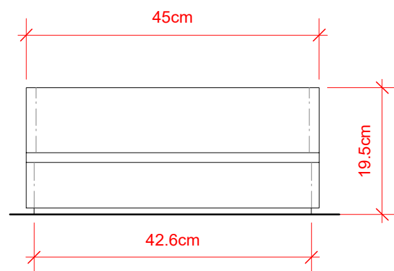
3 Vista Lateral Scale: 1:8
