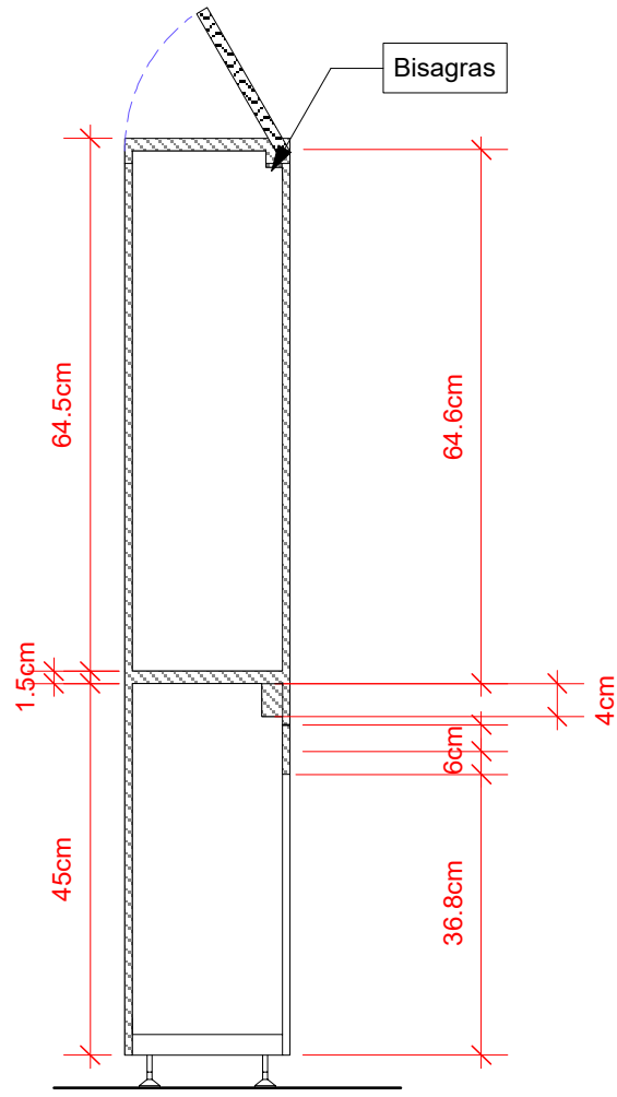
5 Corte Scale: 1:10
