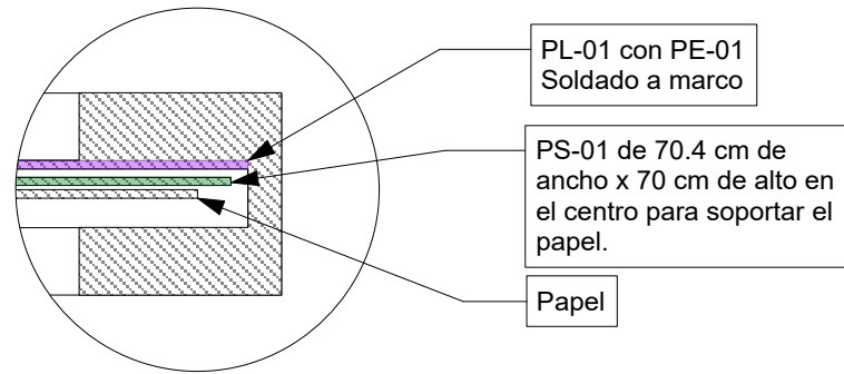
A Corte Scale 2:1
