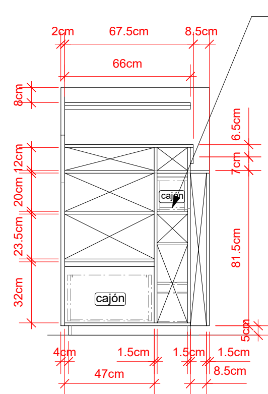
2 Vista Frontal Scale: 1:20
