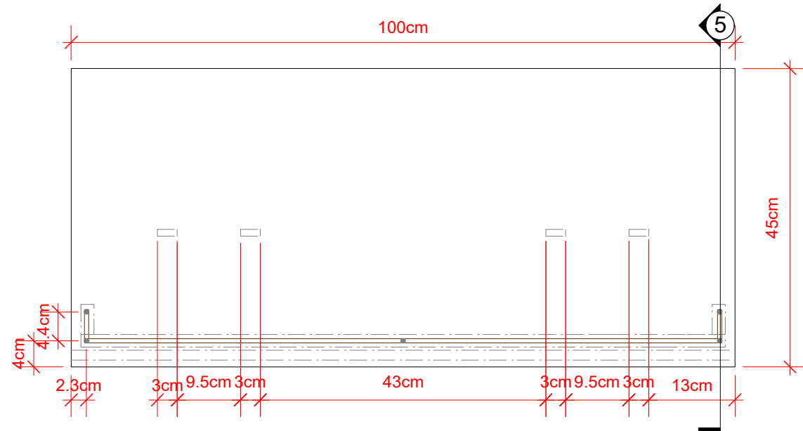
1 Vista Superior Scale: 1:8
