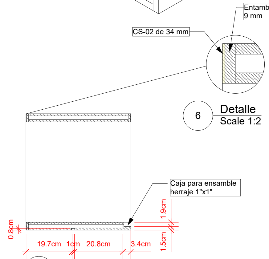
5 Corte Scale: 1:10
