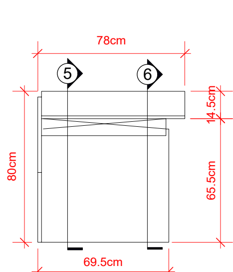
1 Vista Superior Scale: 1:20
