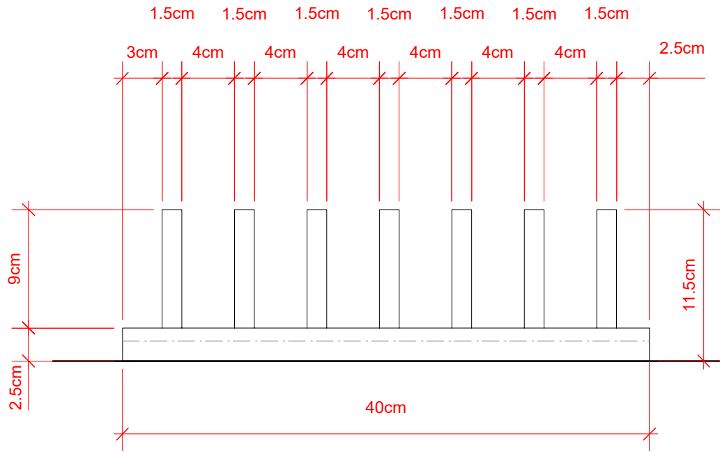
4 Vista Lateral Scale: 1:4
