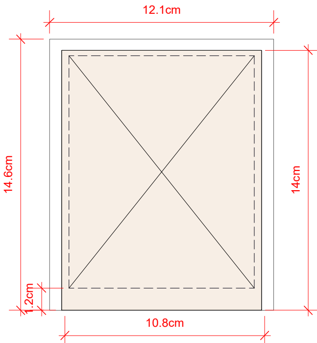
4 Tamaño PS & Papel Scale 1:2
