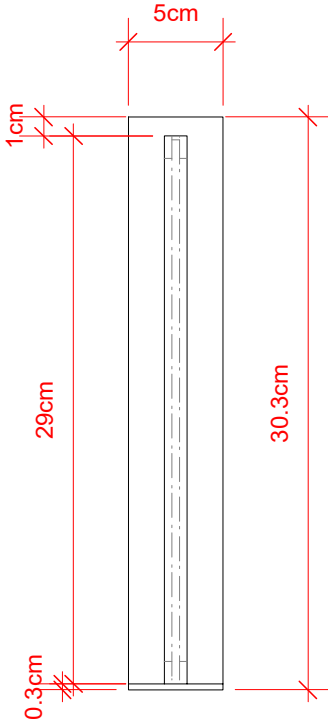
3 Vista Lateral Scale: 1:4
