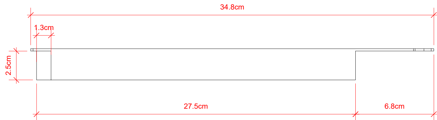
1 Vista Superior Scale 1:2
