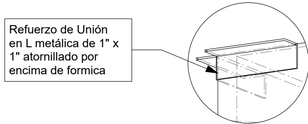
5 Vista desde abajo Isométrico
