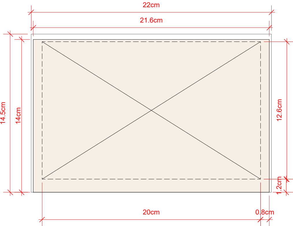
5 Tamaño PS & Papel Scale 1:2
