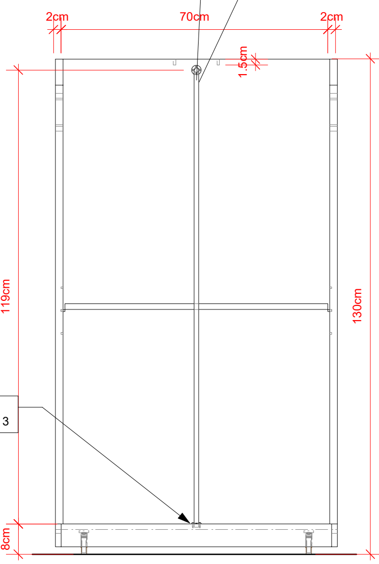
4 Vista Lateral Scale: 1:10
