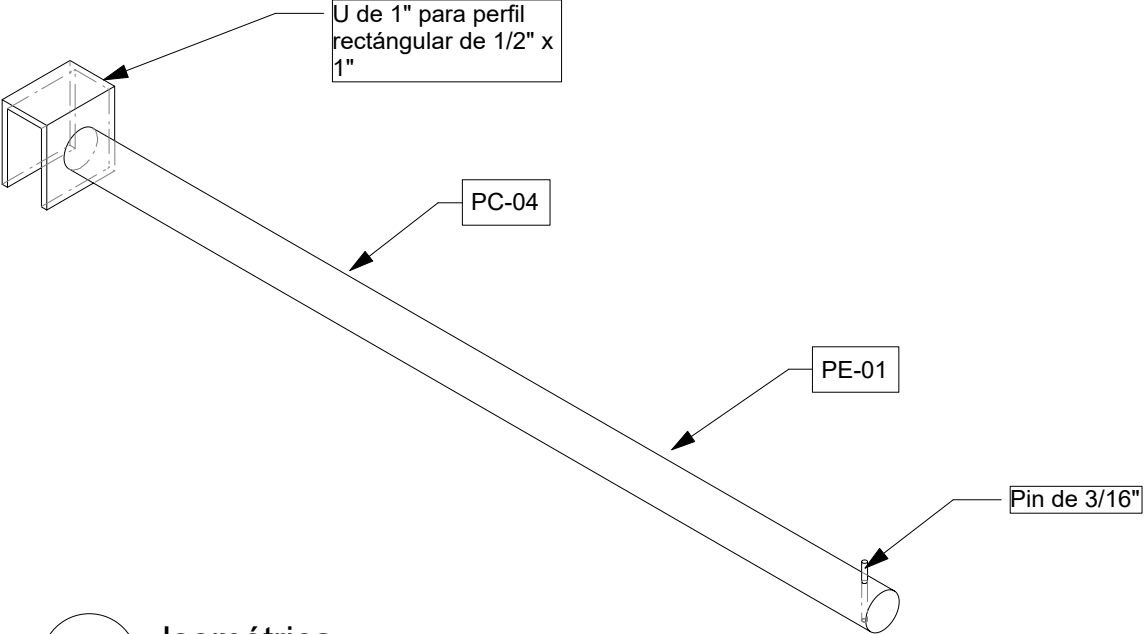
3 Isométrica Scale 1:2
