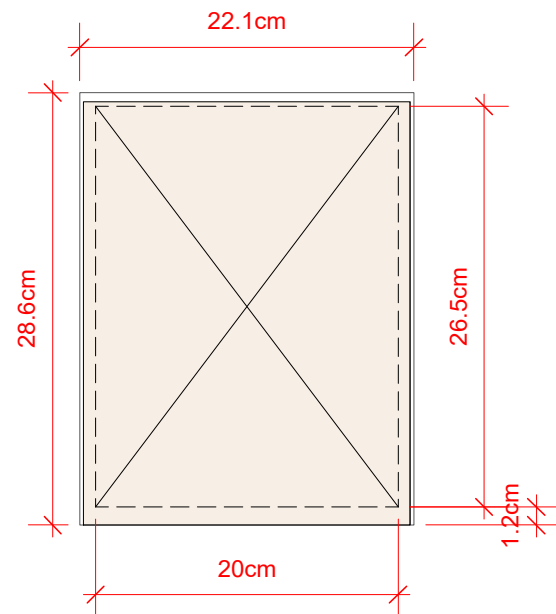
4 Tamaño PS & Papel Scale 1:2
