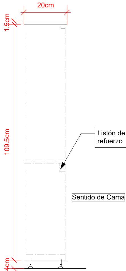
4 Vista Lateral Scale: 1:10
