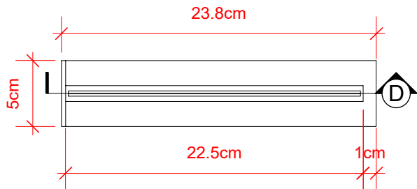
1 Vista Superior Scale: 1:4
