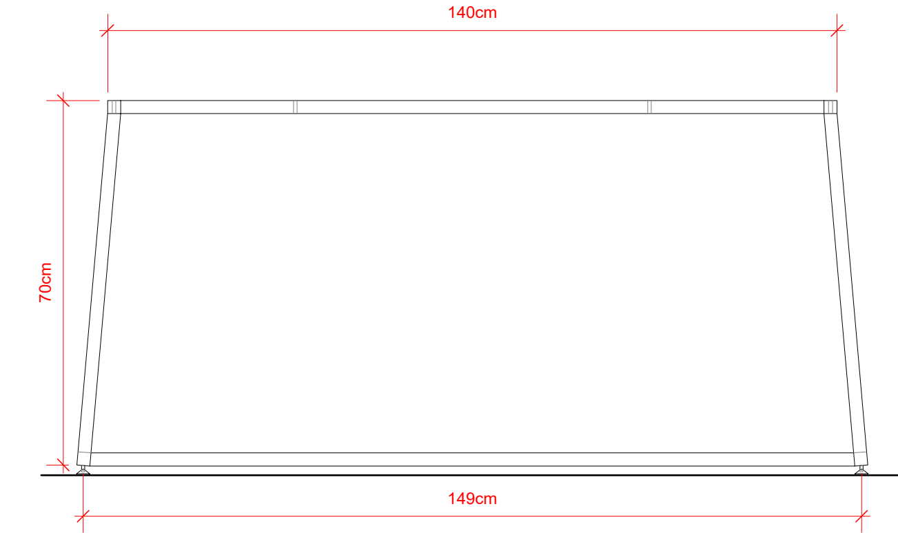
2 Vista Frontal Scale: 1:10
