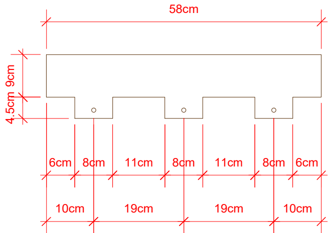
7 Desarrollo Acrílico Scale: 1:8
