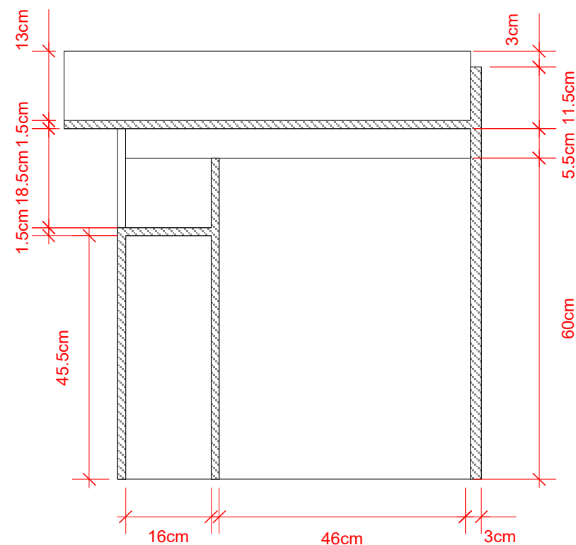
2 Corte C Scale: 1:10
