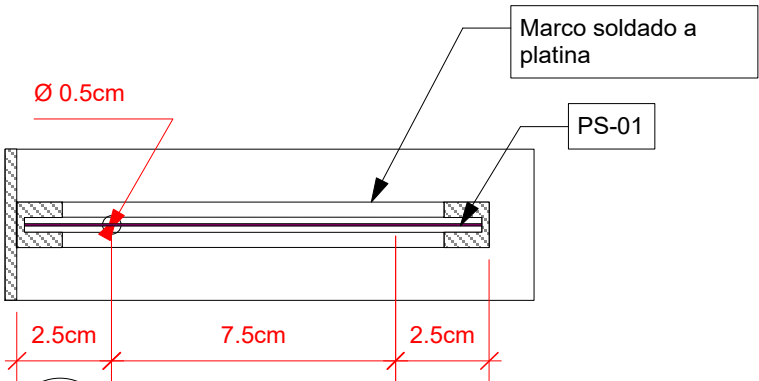
A Corte Scale 1:2
