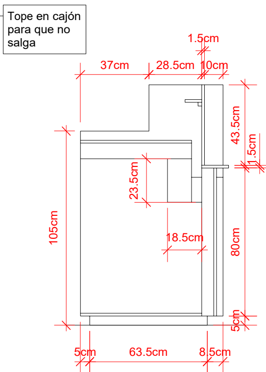
4 Vista Lateral Scale: 1:20
