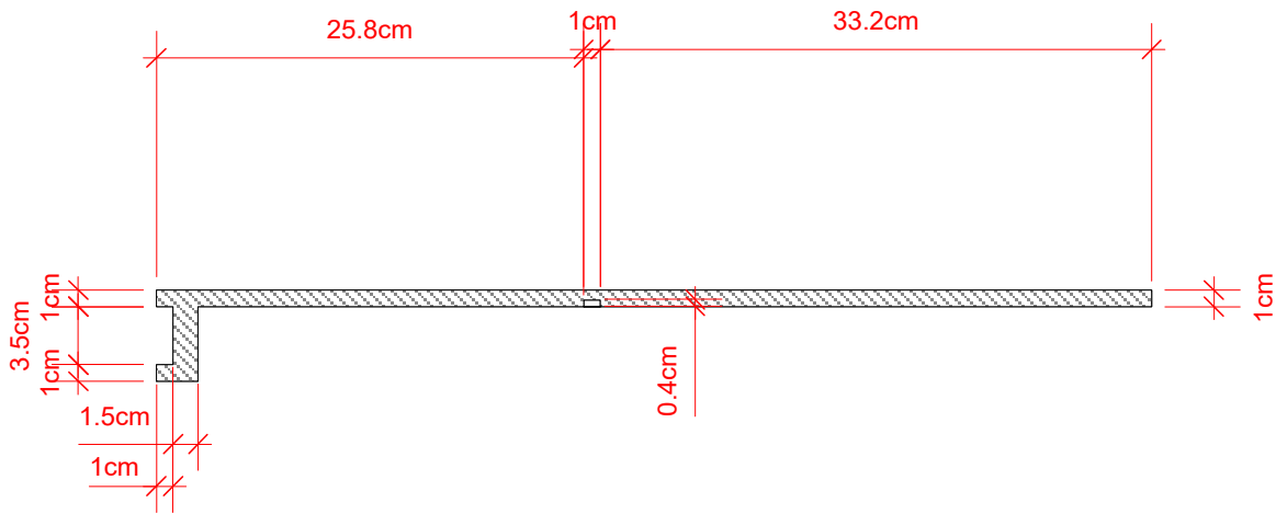
4 Corte Scale: 1:5
