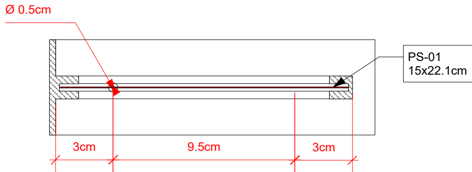
A Corte Horizontal Scale 1:2
