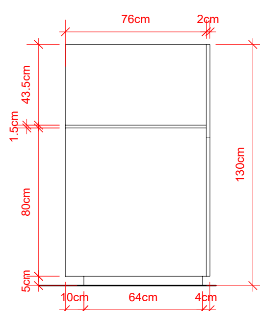
3 Vista Frontal Scale: 1:20
