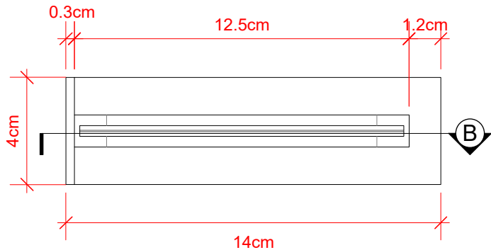
1 Vista Superior Scale 1:2
