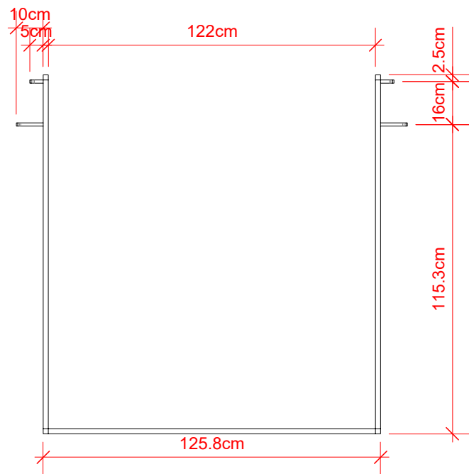
4 Vista Frontal Estructura Scale: 1:20
