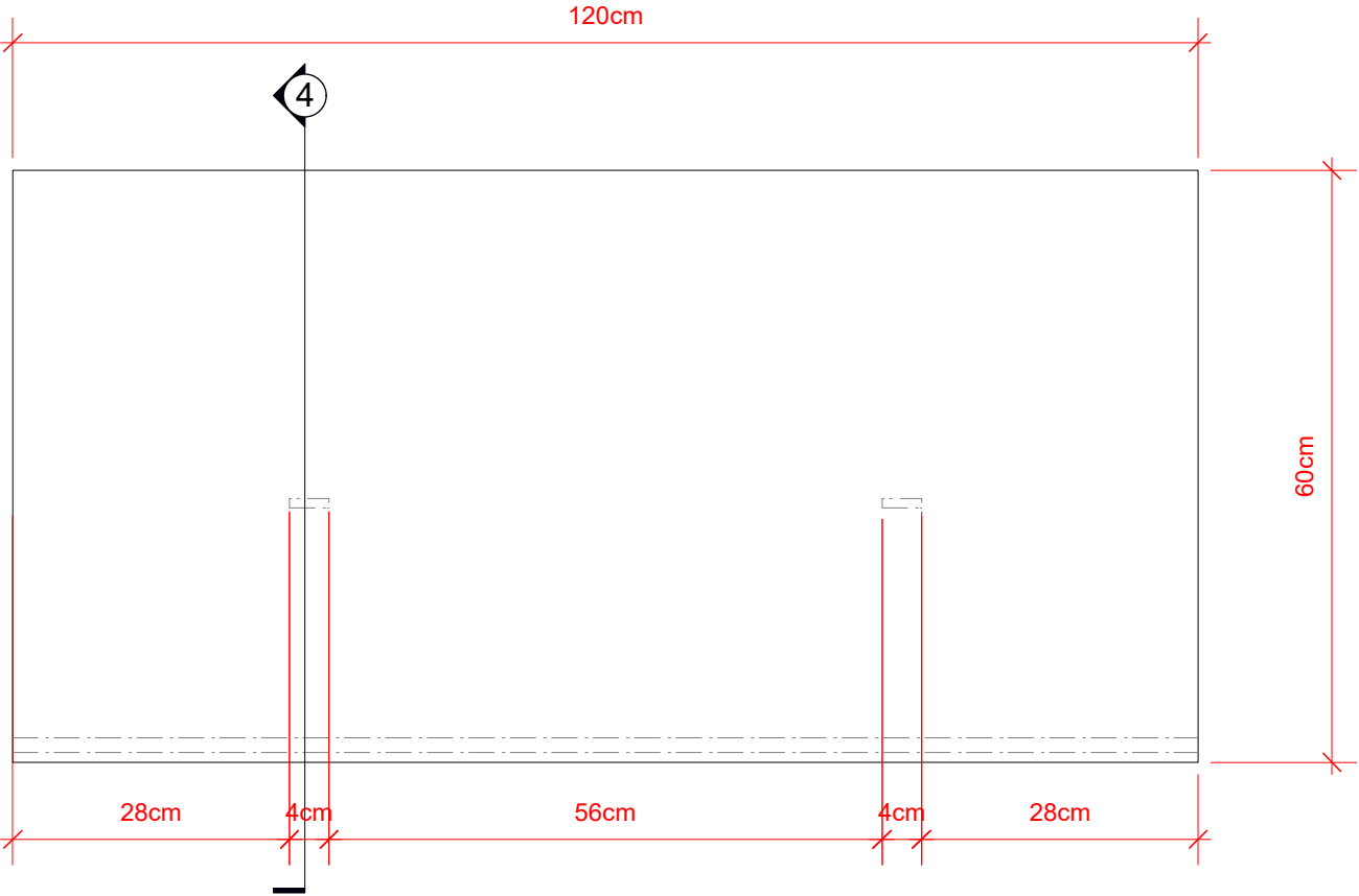
1 Vista Superior Scale: 1:8
