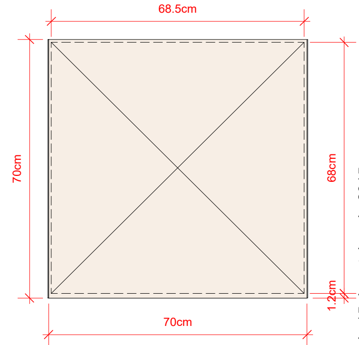
5 Tamaño PS & Papel Scale: 1:10
