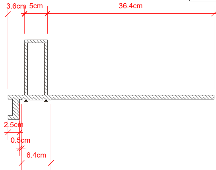
5 Corte Scale: 1:5
