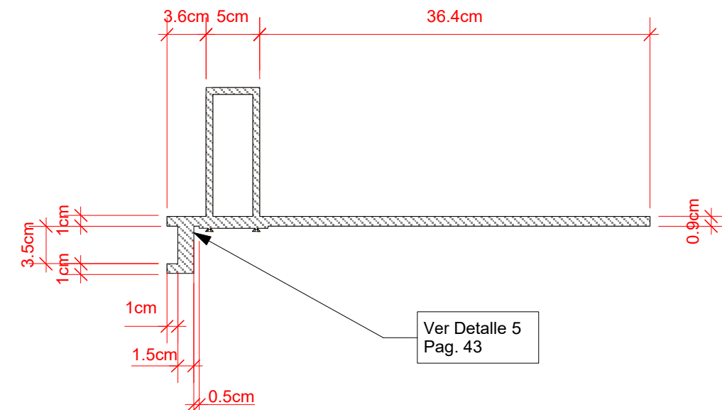
5 Corte Scale: 1:5
