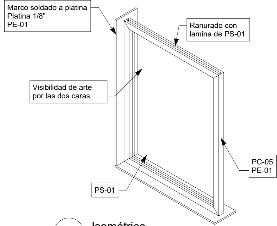
5 Isométrico Scale: 1:4
