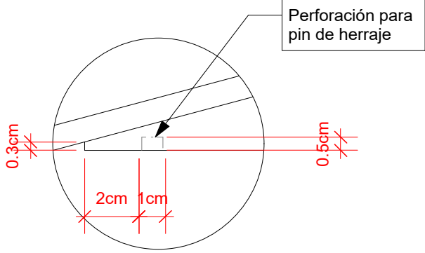
7 Desarrollo Acrílico Scale: 1:8
