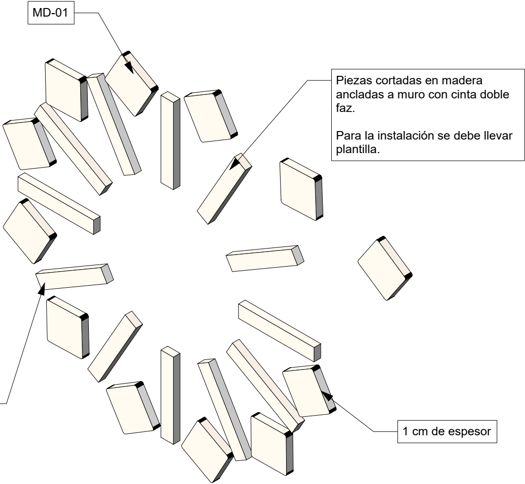
2 Isométrico Scale 1:1
