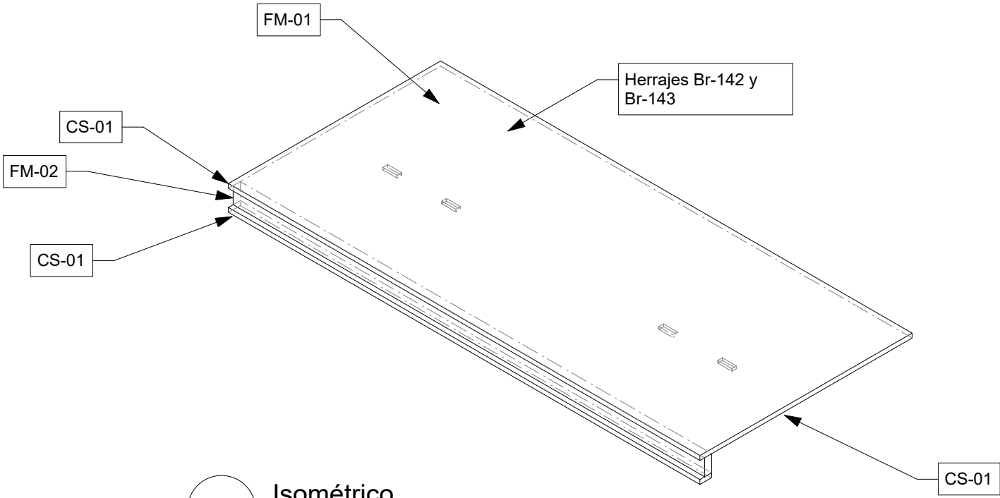
3 Isométrico Scale: 1:8
