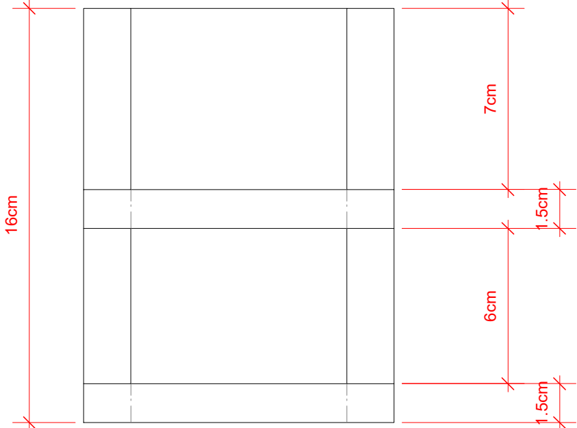
1 Vista Superior Scale 1:2
