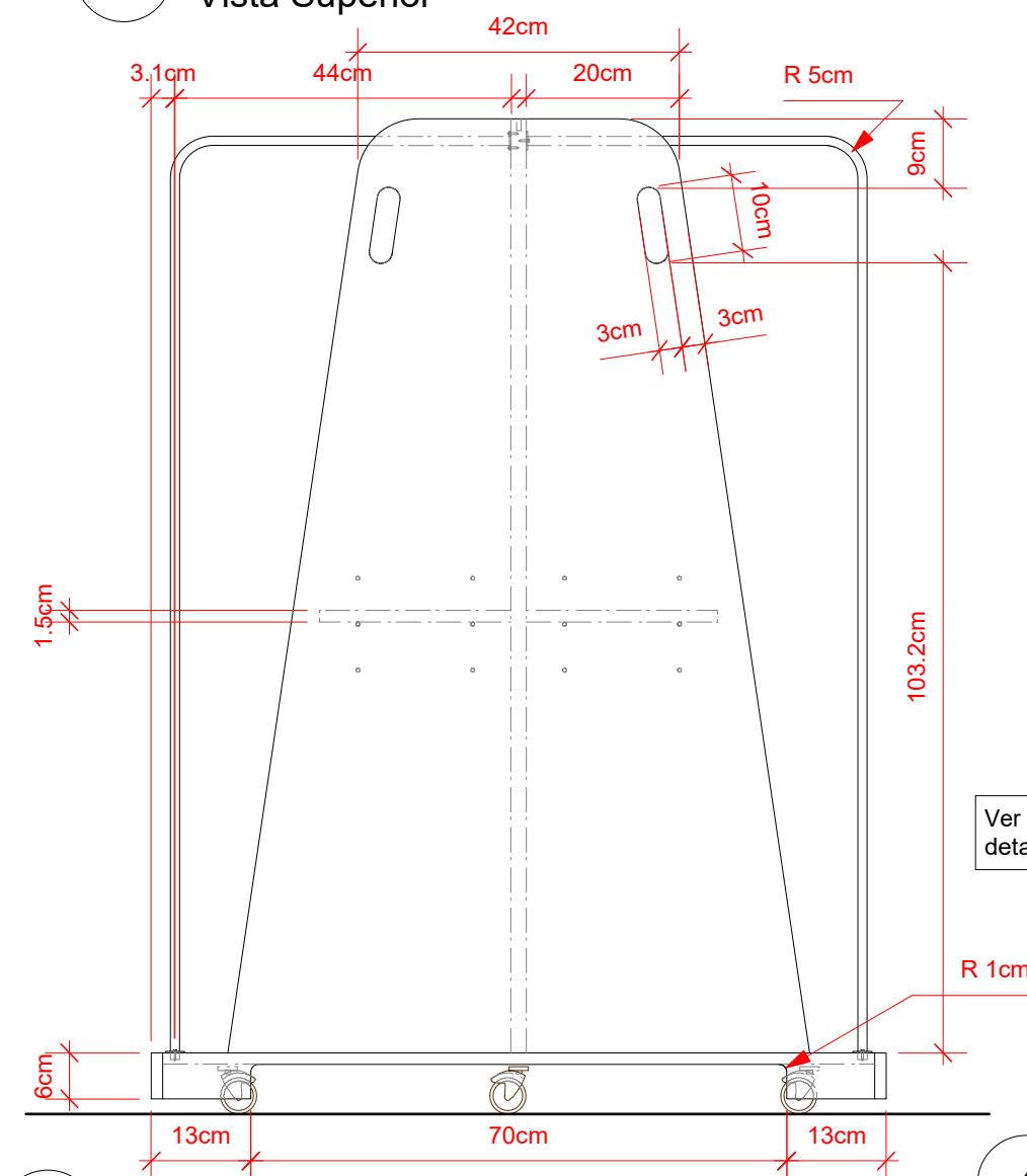
2 Vista Frontal Scale: 1:10
