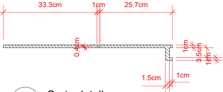
4 Corte detalle Scale: 1:8
