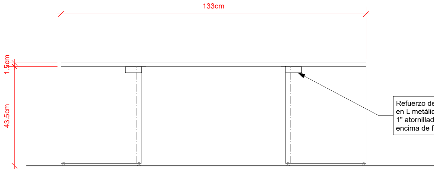
2 Vista Frontal Scale: 1:10
