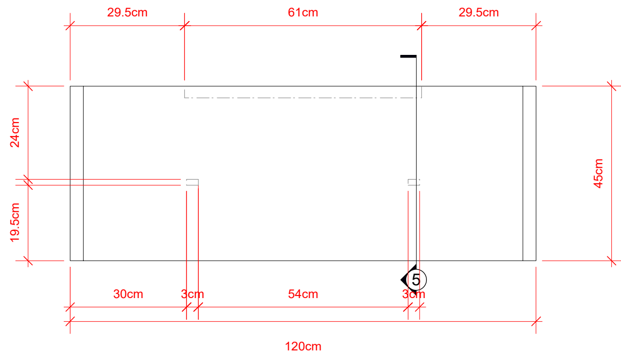
1 Vista Superior Scale: 1:10
