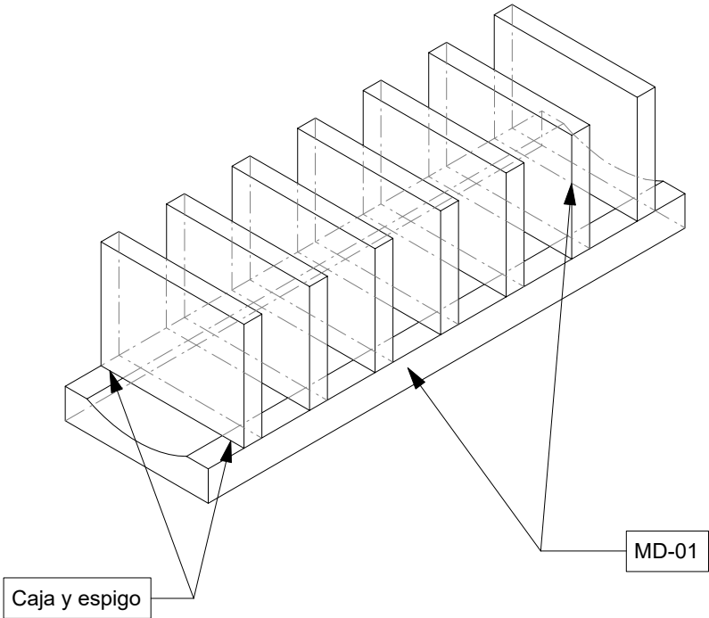
3 Isometrico Scale: 1:4
