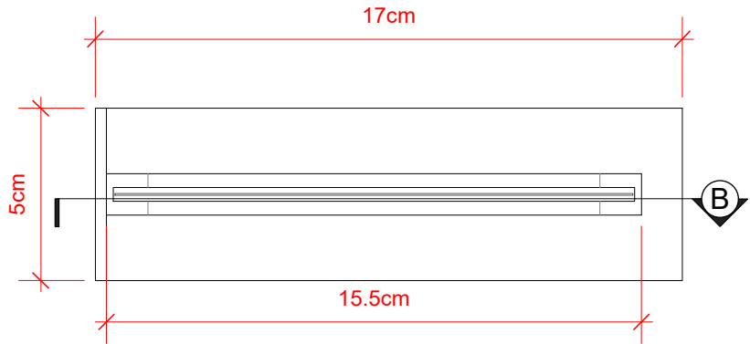
1 Vista Superior Scale 1:2
