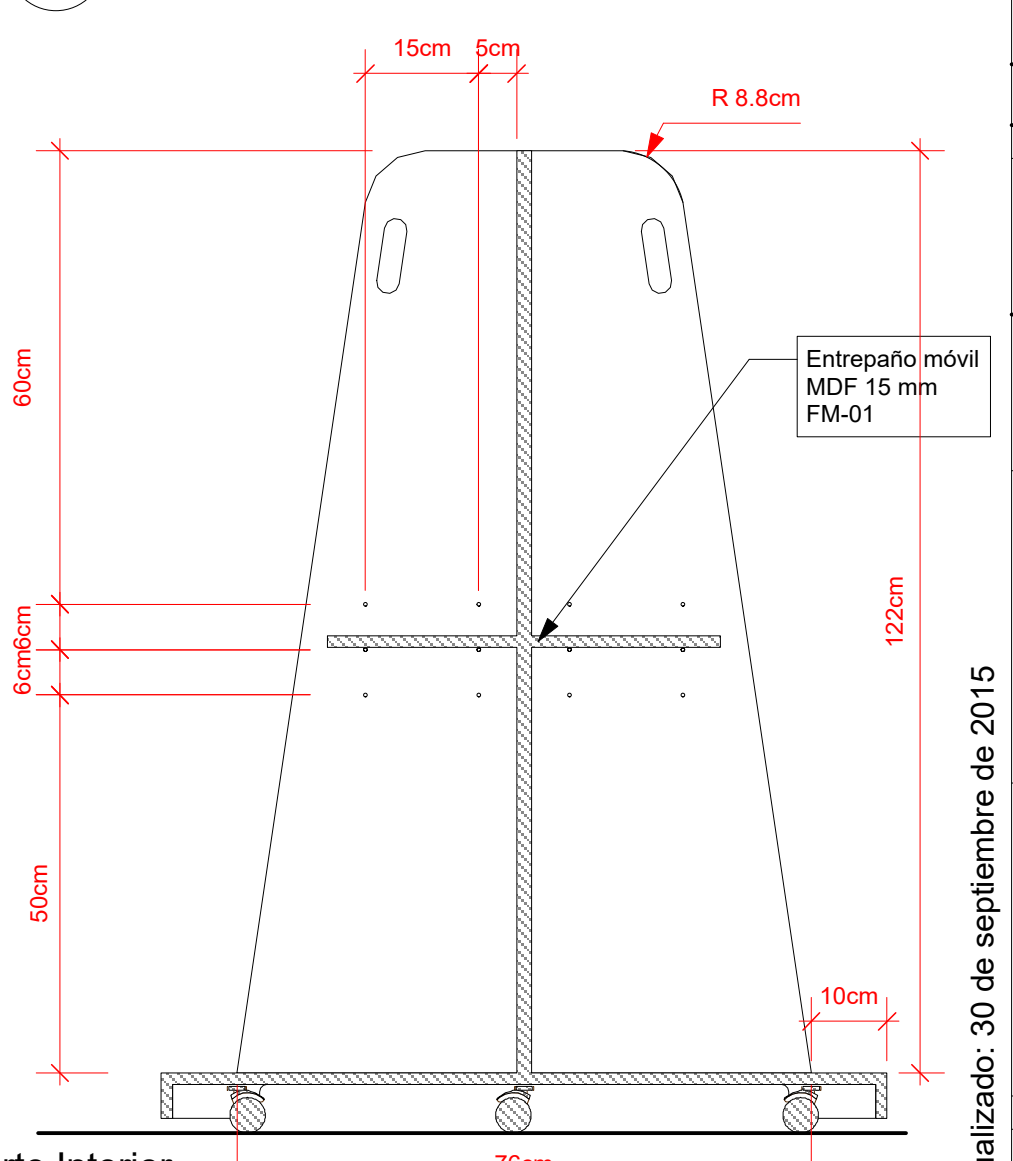
7 Corte Interior Scale: 1:10
