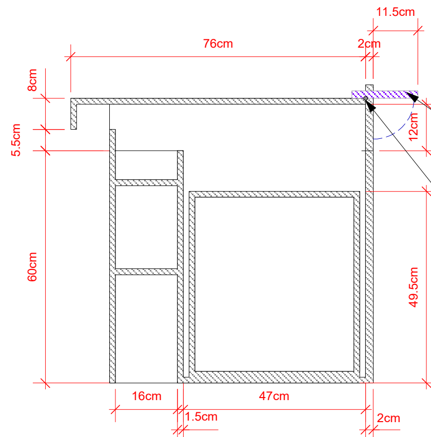
4 Corte D Scale: 1:10
