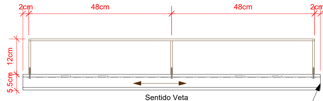
2 Vista Frontal Scale: 1:8
