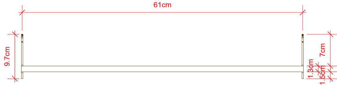
1 Vista Superior Scale: 1:5
