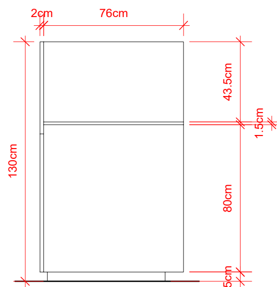
5 Vista Frontal Scale: 1:20
