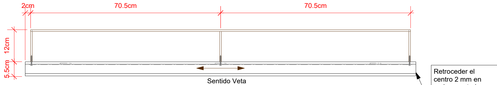
2 Vista Frontal Scale: 1:8
