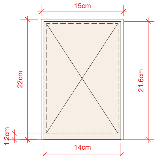
4 Tamaño PS & Papel Scale: 1:4
