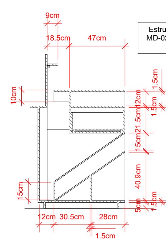
6 Corte B Scale: 1:20
